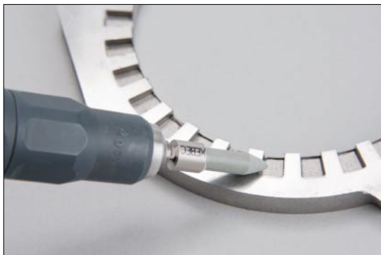
エッジ部バリ取り
