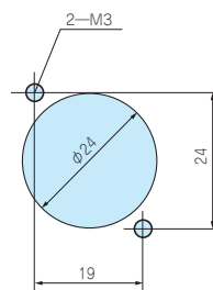
●コネクタ取付穴寸法図
