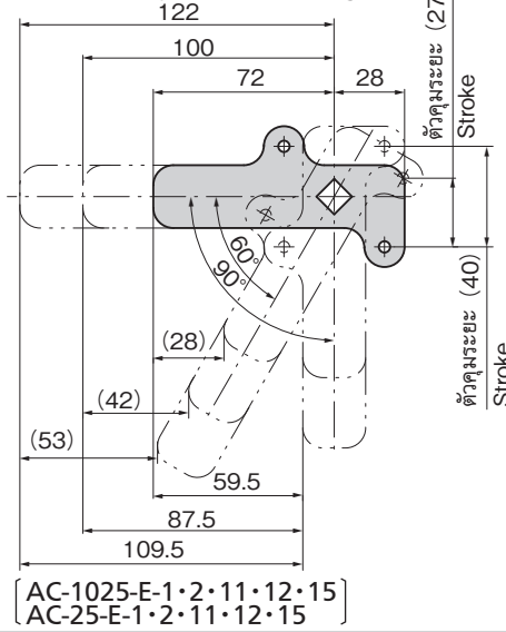
แผนภาพการทำงาน Operation drawings
