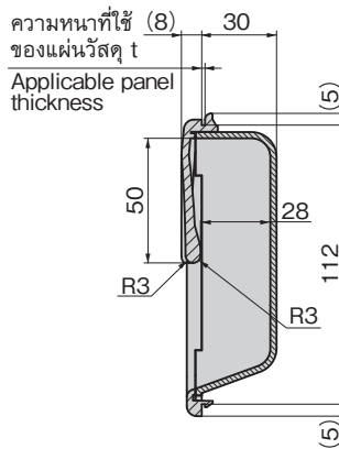
ด้านตัด A-A A-A section
