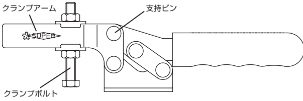
○最大力量のクランプボルト位置
