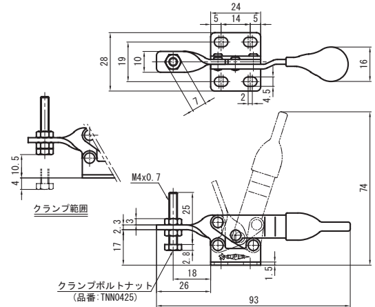
○最大クランプ範囲のクランプボルト位置
