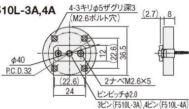
外形寸法図
