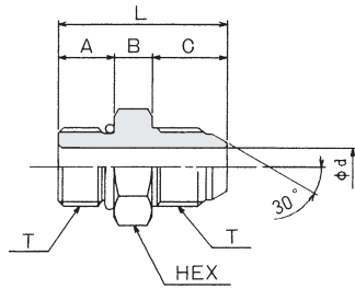
接続口金具 : SR-04
