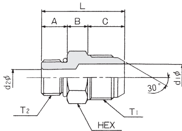
接続口金具 : SR-04
