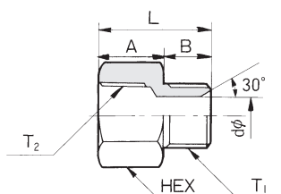
接続口金具 : SR-01・SR-05
