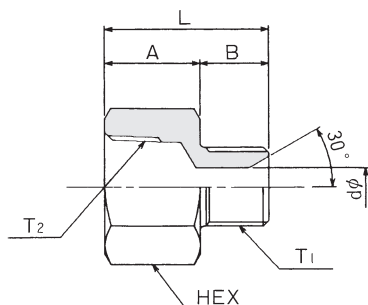
接続口金具 : SR-01・SR-05
