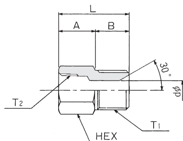
接続口金具 : SR-01・SR-05
