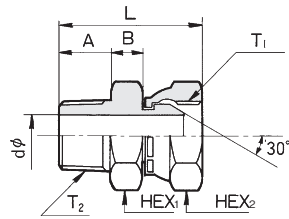
接続口金具 : SR-02
