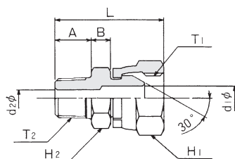
接続口金具 : SR-02
