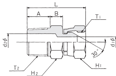
接続口金具 : SR-02
