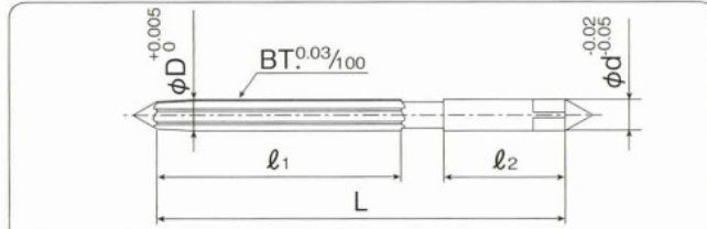
食付き角 1^\circ 1° Chamfer ※図は \phi 3.0 未満の形状です。 Figure is shape of less than \phi 3.0
