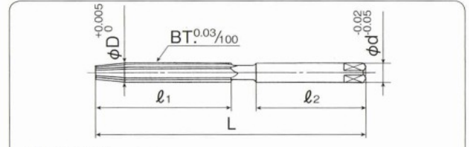
食付き角 1^\circ 1° Chamfer ※図は \phi 3.0 以上の形状です。 Figure is shape of \phi 3.0 or more
