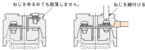
(圧着端子締付例)
