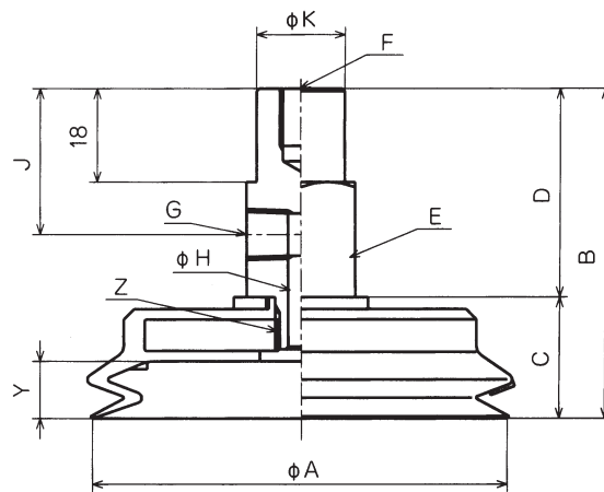
PJYK-60/70/80
