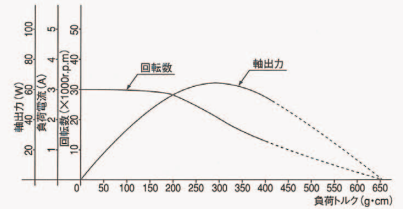
● 特性曲線
