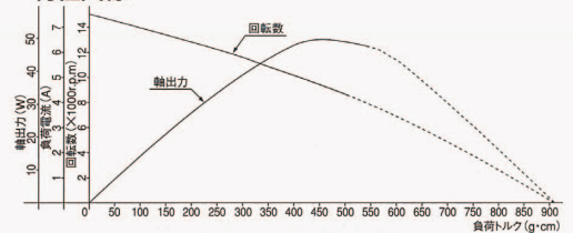
● 特性曲線
