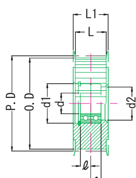
(TPI-150H~TPI-200H)
