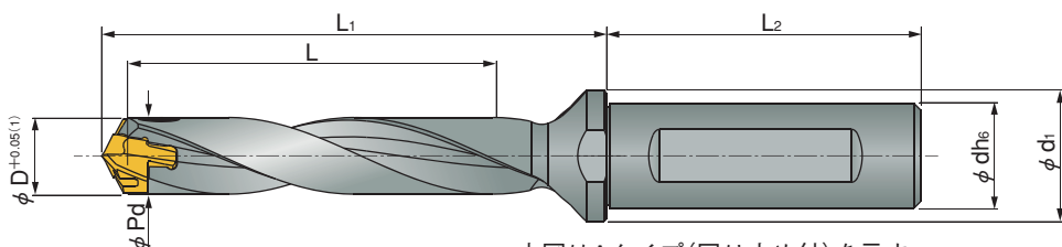
本図はAタイプ(回り止め付)を示す。
