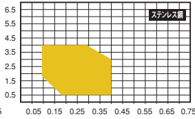
WNMG 080408-VL
