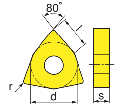
WNMG 080408-WG
