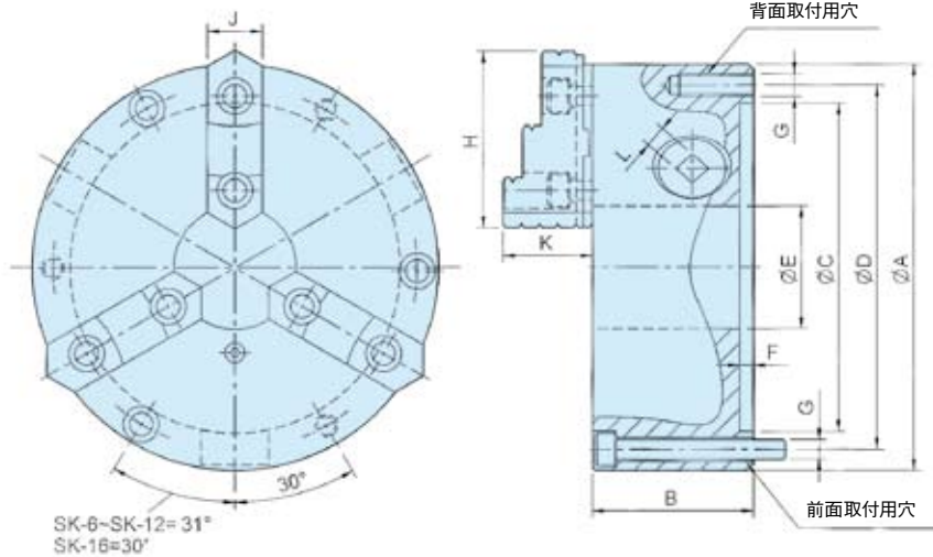
前面取付仕様 / 前面・背面取付兼用仕様
