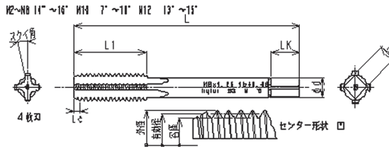
適用範囲 ハンドタップ M6～M12 オーバーサイズハンドタップ M6～M12
