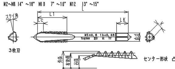
適用範囲 ハンドタップ M2～M5 オーバーサイズハンドタップ M2～M5
